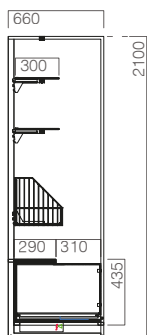
RUP expositor de pão bread wall display
