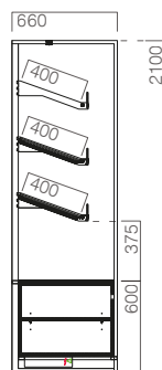
RUB expositor de pão com móvel baixo bread wall display with low cabinet
