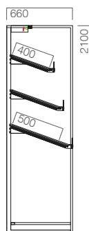
RULSA expositor de pão para autosserviço self-service bread wall display
