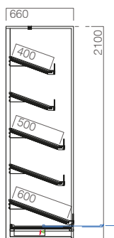
RULS expositor de pão para autosserviço self-service bread wall display
