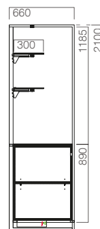
RUC expositor com móvel de serviço wall display with service counter
