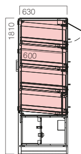
RUACP expositor aquecido heated display DIM. 937
