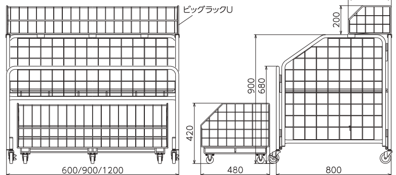
ビッグワゴンU
