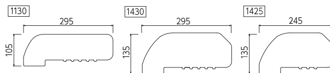
スリットボックス仕切り板
