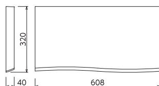
みやびステージ6032 新サイズ
