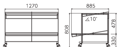
ワイヤー産直什器120
