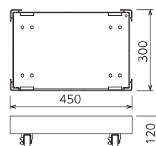
プロモーションラックベース
