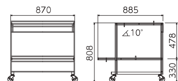
ワイヤー産直什器90
