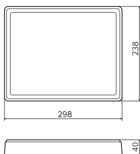
炭火焼鳥トレー30S
