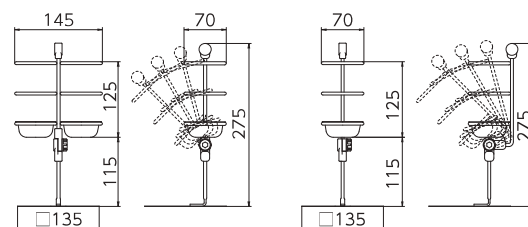
トングスタンドH型
