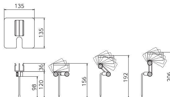
トングスタンドC型SC
