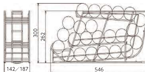
缶オートフェースラック
