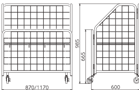
ビッグワゴンA
