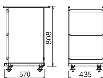
インナーカート
