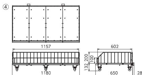
ジャンブルキャリーP60120
