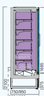
MF2 700/900 N CP FV - CG 3L1 (-18...-15 °C) dim. 1562 | 2343 | 3124 (1)
