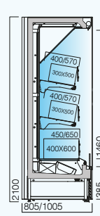
MF2 700/900 PF CC - CG 3H1 (+1...+10 °C) dim. 1250 | 1562 | 1875 | 2500 (1) | 3750 (1)
