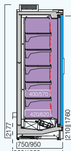
MF2 700/900 N CP FV - CG 3L1 (-18...-15 °C) dim. 1562 | 2343 | 3124 (1)
