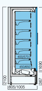
MF2 700/900 P CP FV - CG 3M1 (-1...+5 °C) | 3M2 (-1...+7 °C) dim. (2) 937 | 1250 | 1562 | 1915 (3) | 1875 | 2015 (3) | 2500 (1) | 3750 (1)
