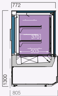
VVSTGL congelados frozen products 6L1 (-24... -20 °C) dim. 850 | 1250
