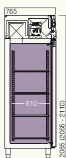
ANXT GN1/1 VN 4L1 (-18...-15 °C) ANXTA5 GN1/1 VN 5L1 (-18...-15 °C) DIM. 5851P
