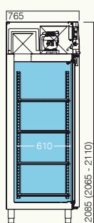
ANXT GN1/1 VP 4M1 (-1...+5 °C) ANXTA5 GN1/1 VP 5M1 (-1...+5 °C) DIM. 5851P
