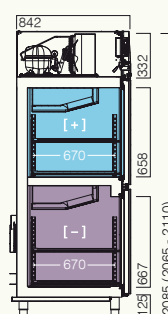
ANXT GN2/1 VM 4M1/4L1 (-1...+5/-18...-15 °C) ANXTA5 GN2/1 VM 5M1/5L1 (-1...+5/-18...-15 °C) DIM. 7302MP | 1460 2P
