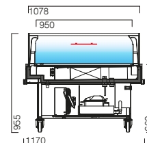
EXPV RV 3M2 ventilada ventilated ventilée ventilada
