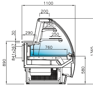
PARPGV 3M2 ventilada com gavetão fan assisted w/ slide-out drawer ventilée avec tiroir ventilada con cajón
